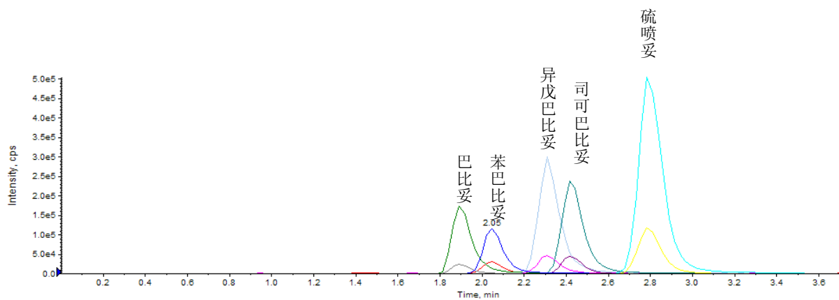
图 B 5 种巴比妥类药物的 MRM 色谱图
